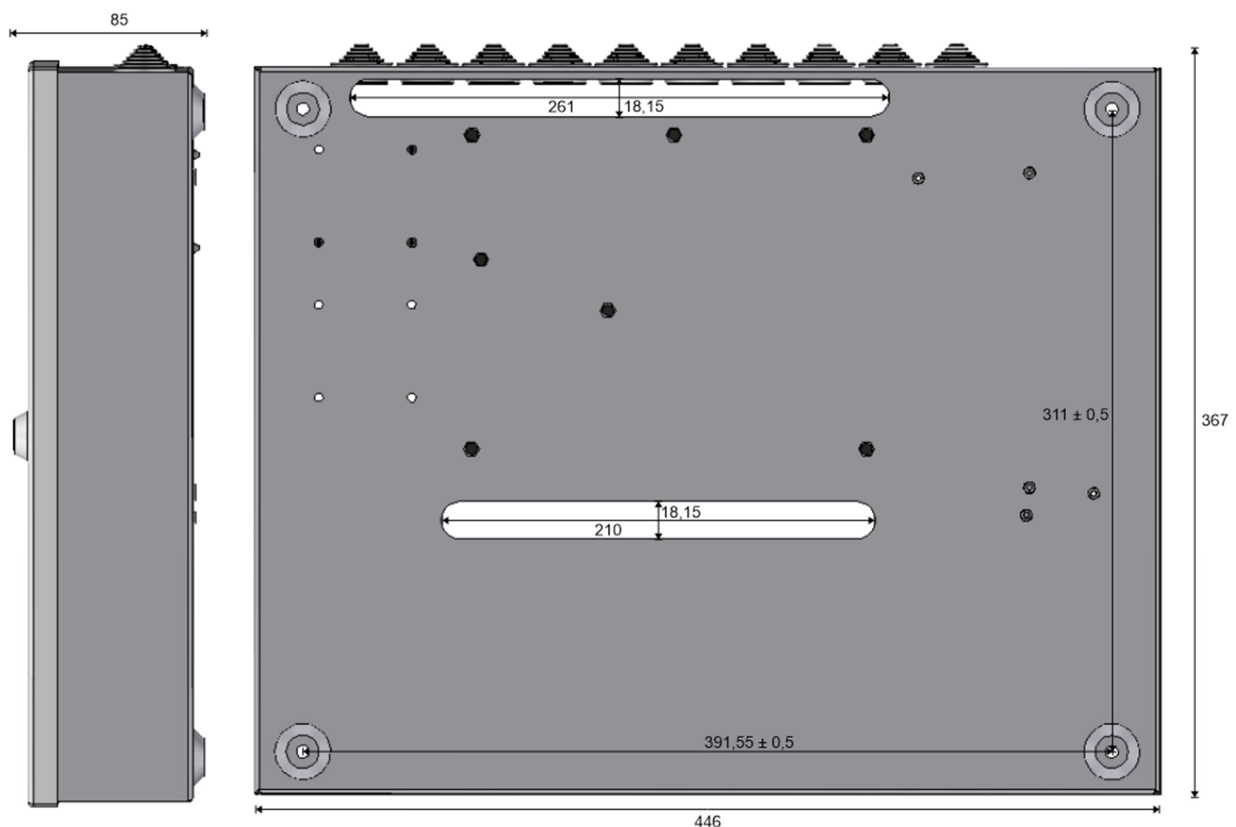
Maßzeichnung (mm):
