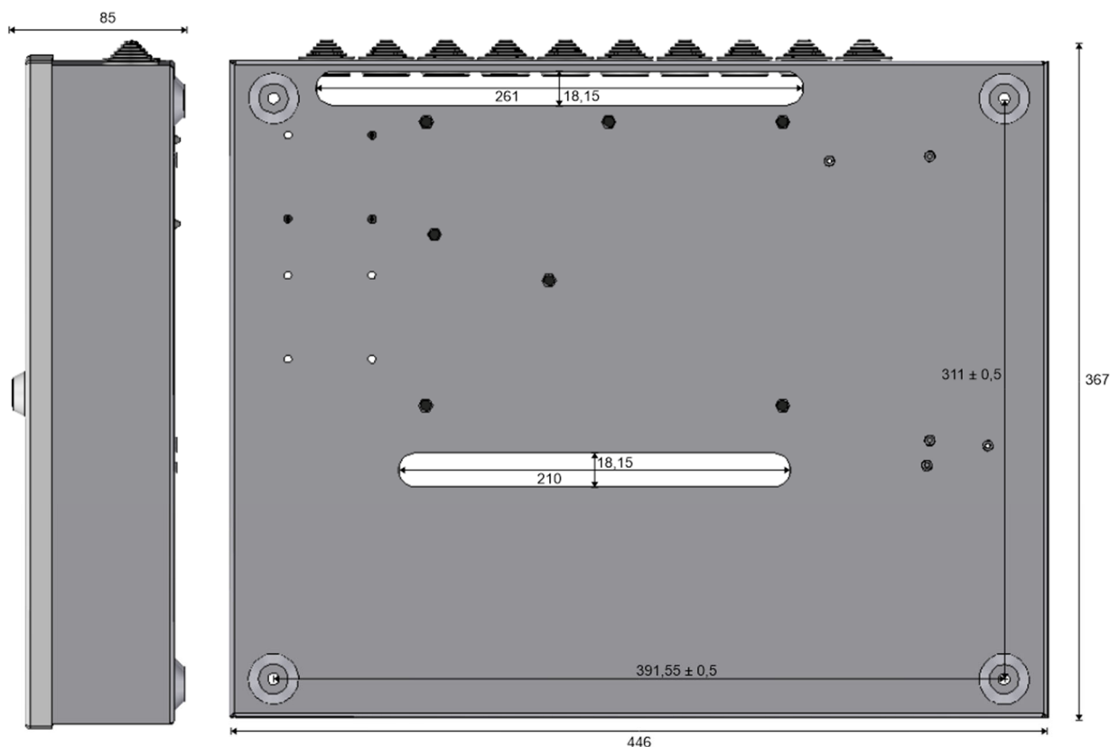
Rysunek wymiarowy (mm):
