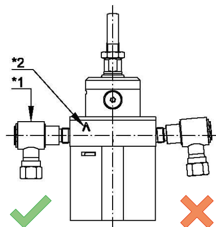
Abbildung 5: Pfeilrichtung
