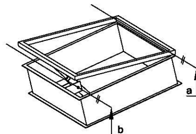
Abbildung 4: Montage
