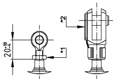
Abbildung 6: Kolbenstangenaufhängung
