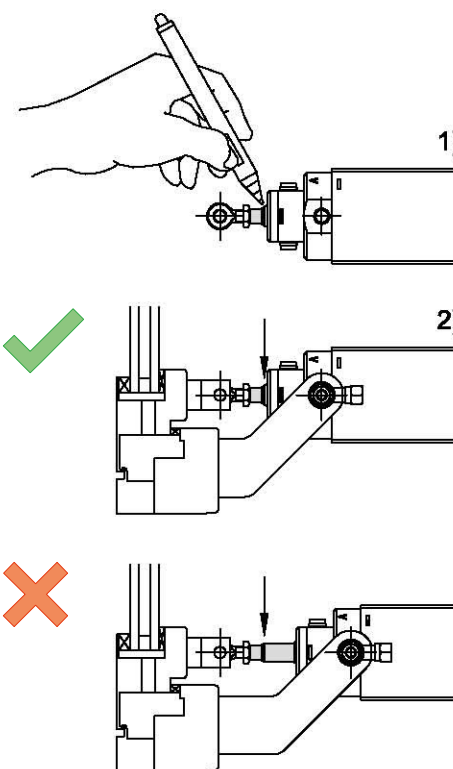
Abbildung 3: Endposition
