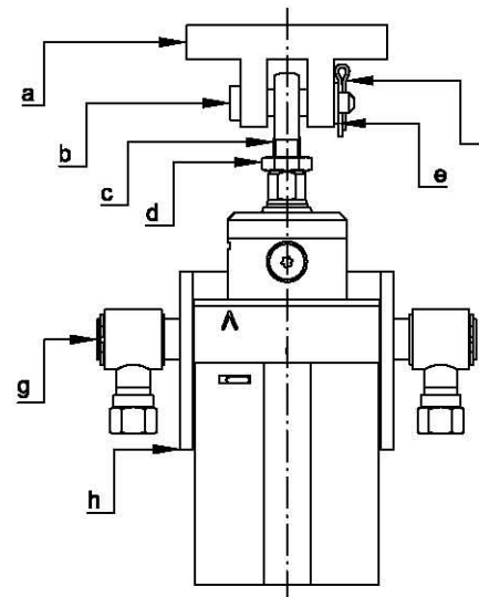
Abbildung 2: Befestigungselemente
