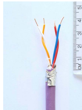
Abschirmung und Beidraht um die Leitung wickeln
