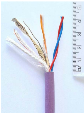
Bus-Leitung abmanteln
